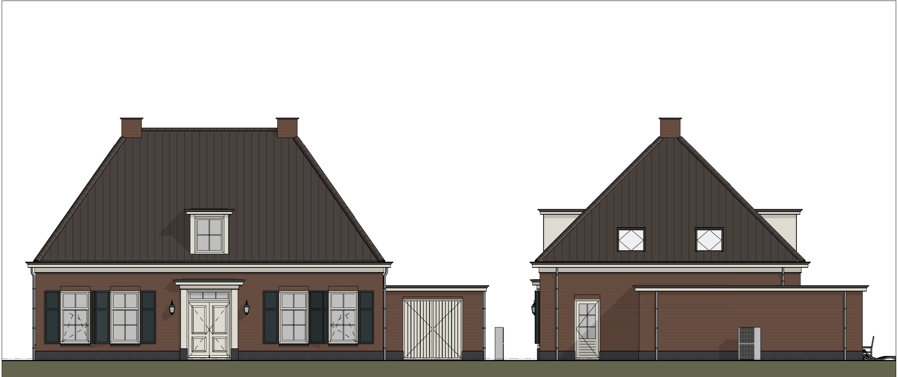
voorgevel
